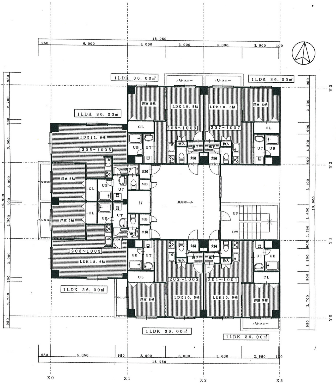
2~10階平面図
