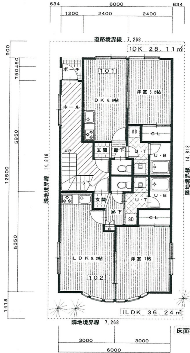
配置図 1階平面図
