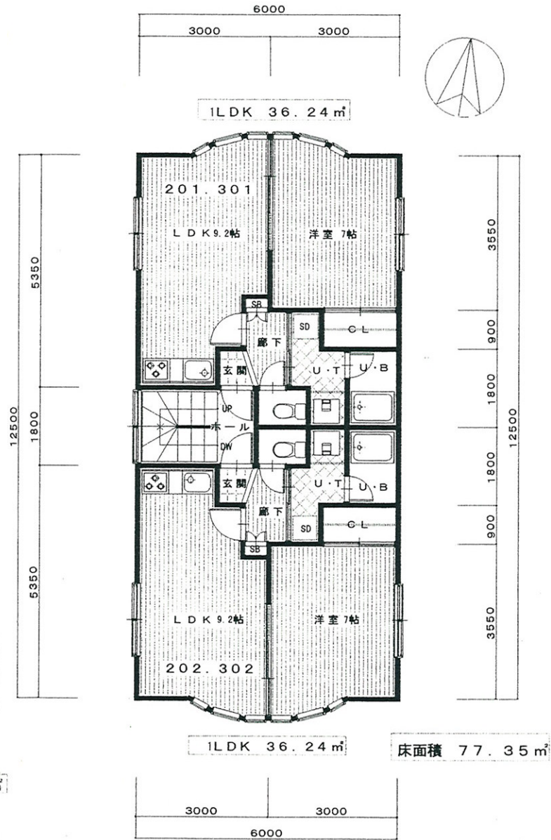
2.3階平面図
