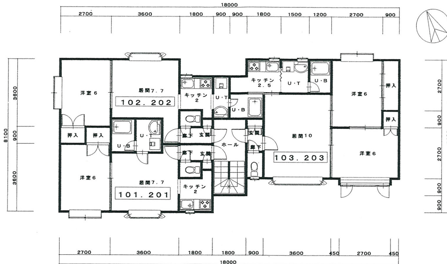
フォーサイトロイヤル 2.3階 平面図
