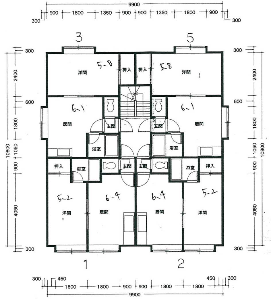
1階・2階平面図
