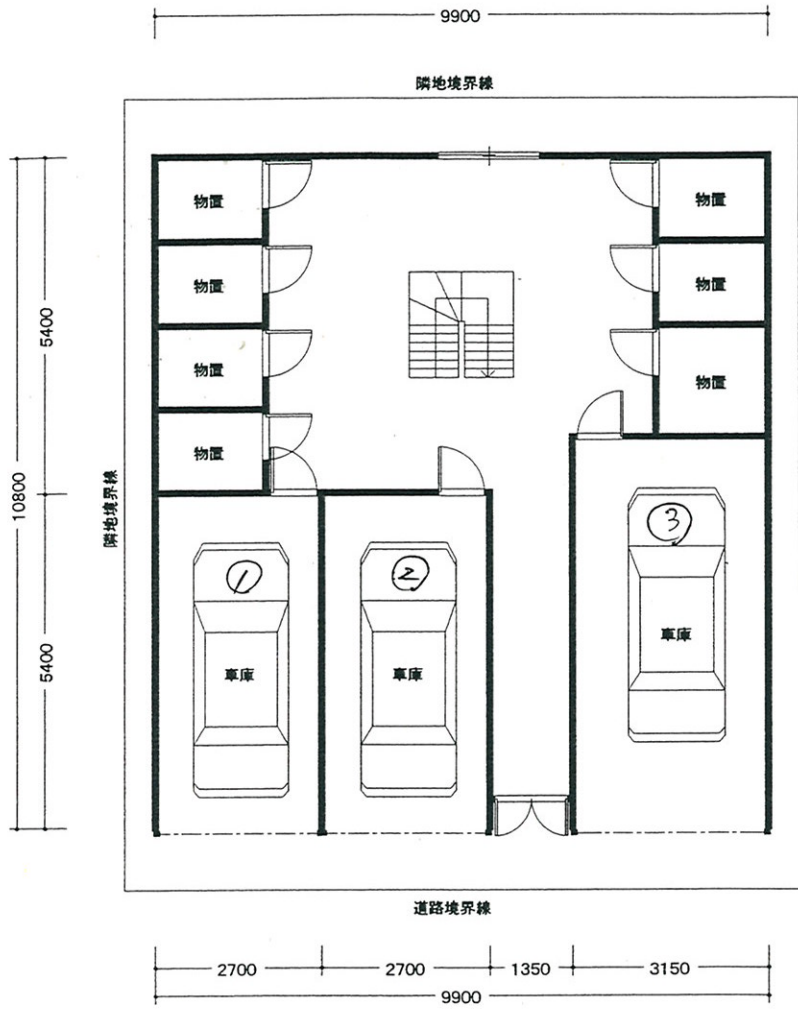
地階平面図
