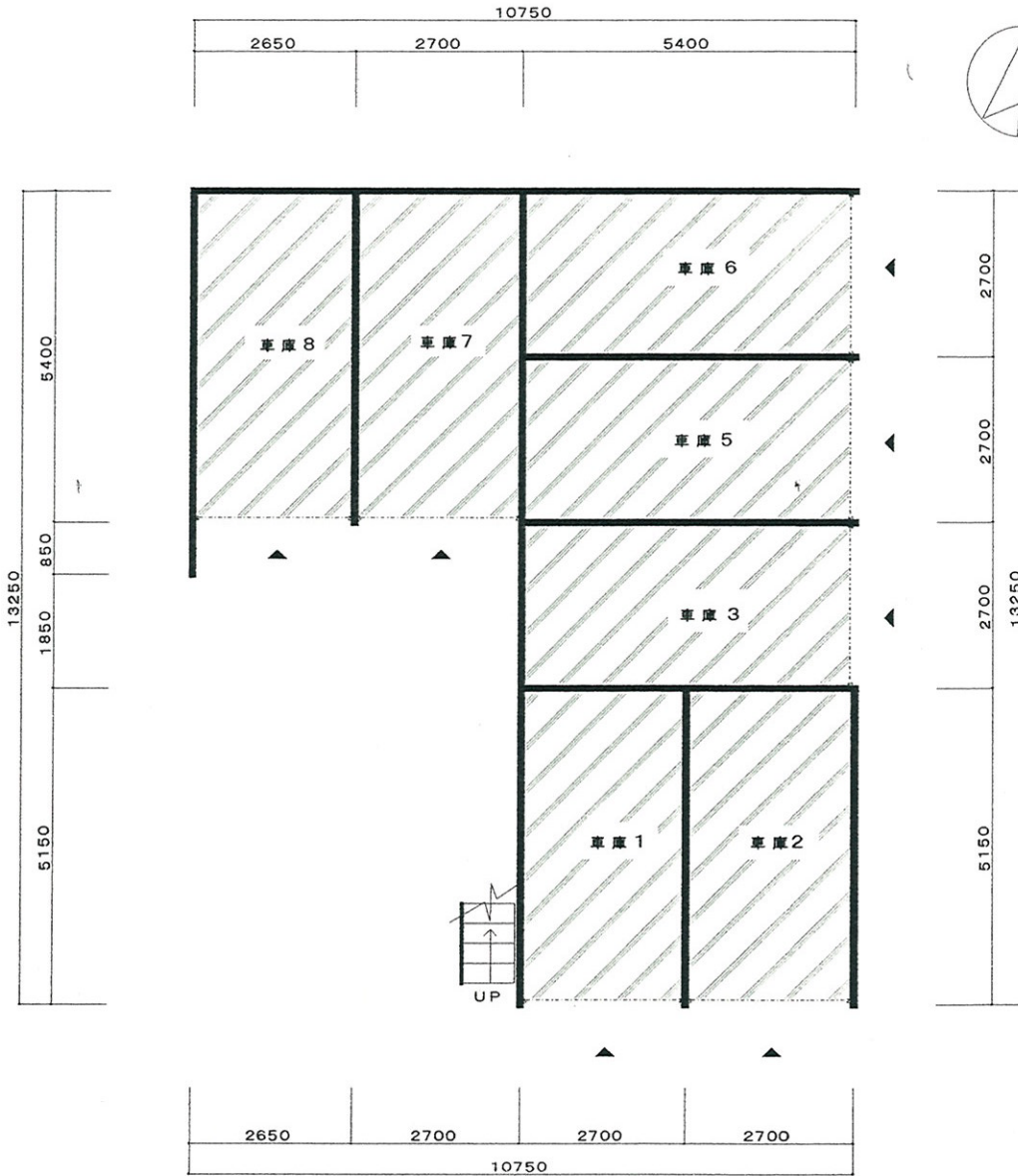
CH創成 A棟 地階平面図
