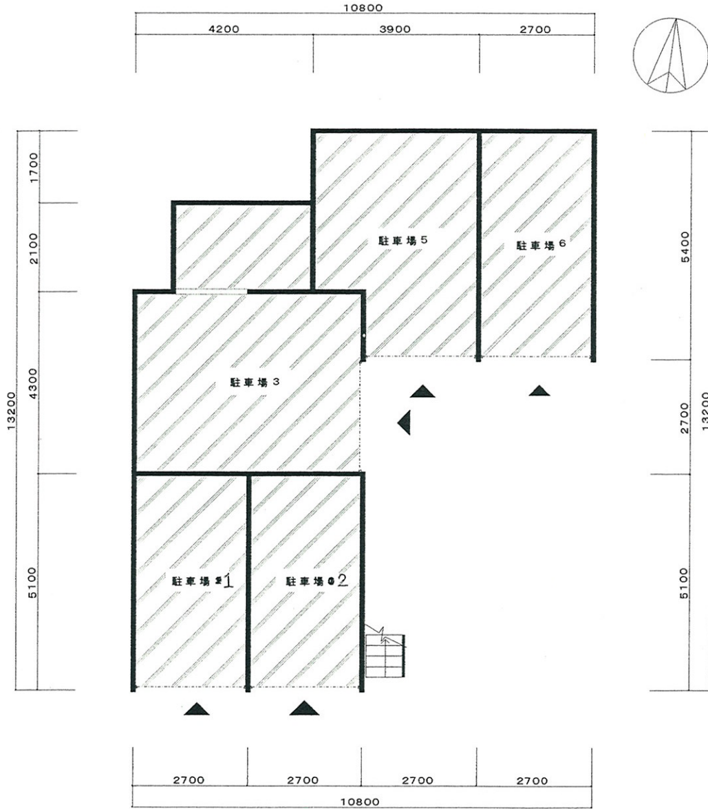
CH創成B棟 地階平面図
