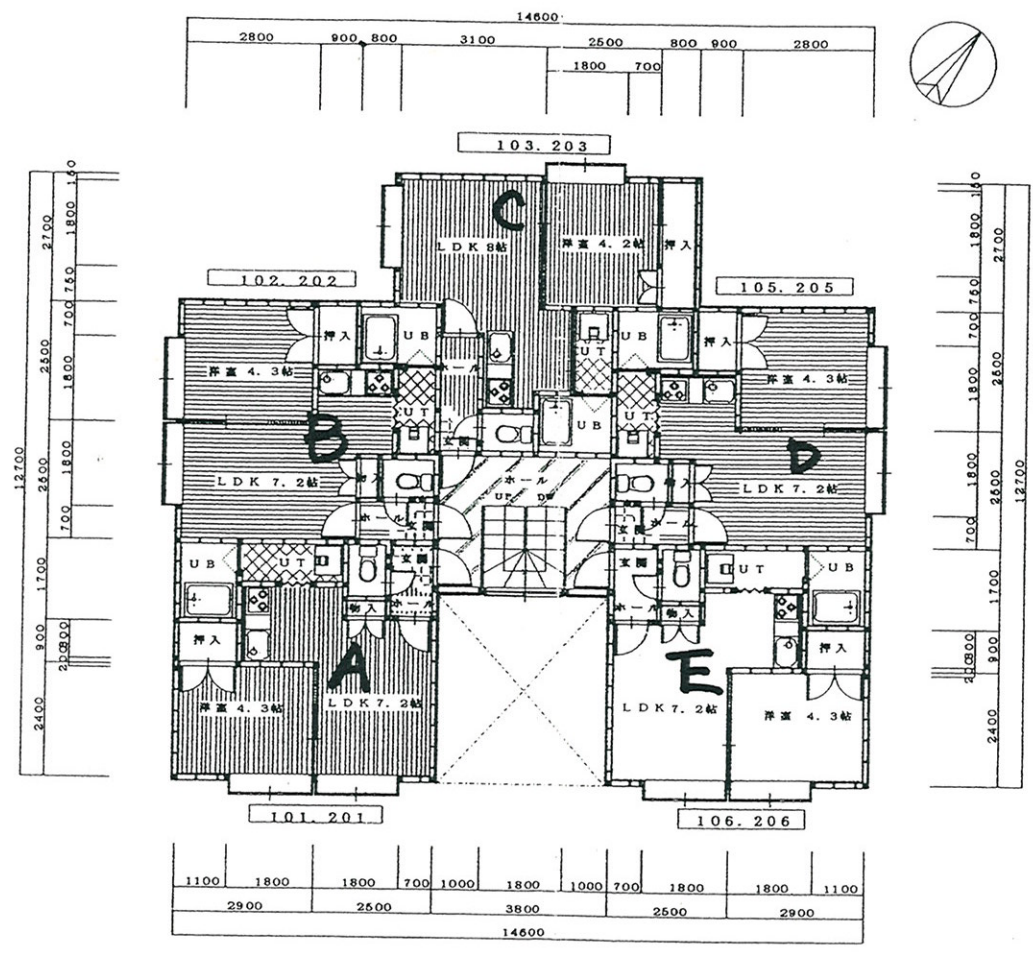
2.3.階平面図
