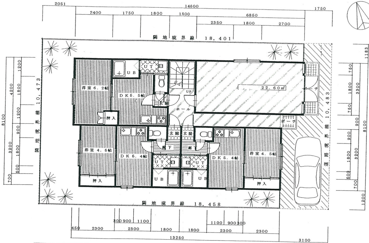
配置図 1階平面図
