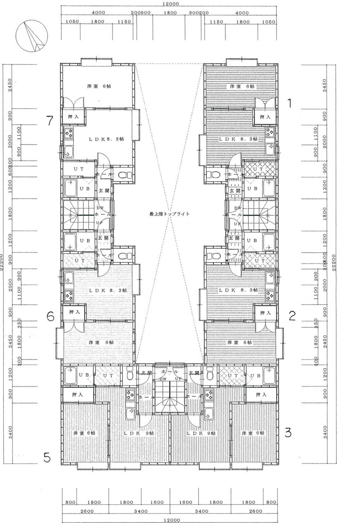
2. 3階 平面図
