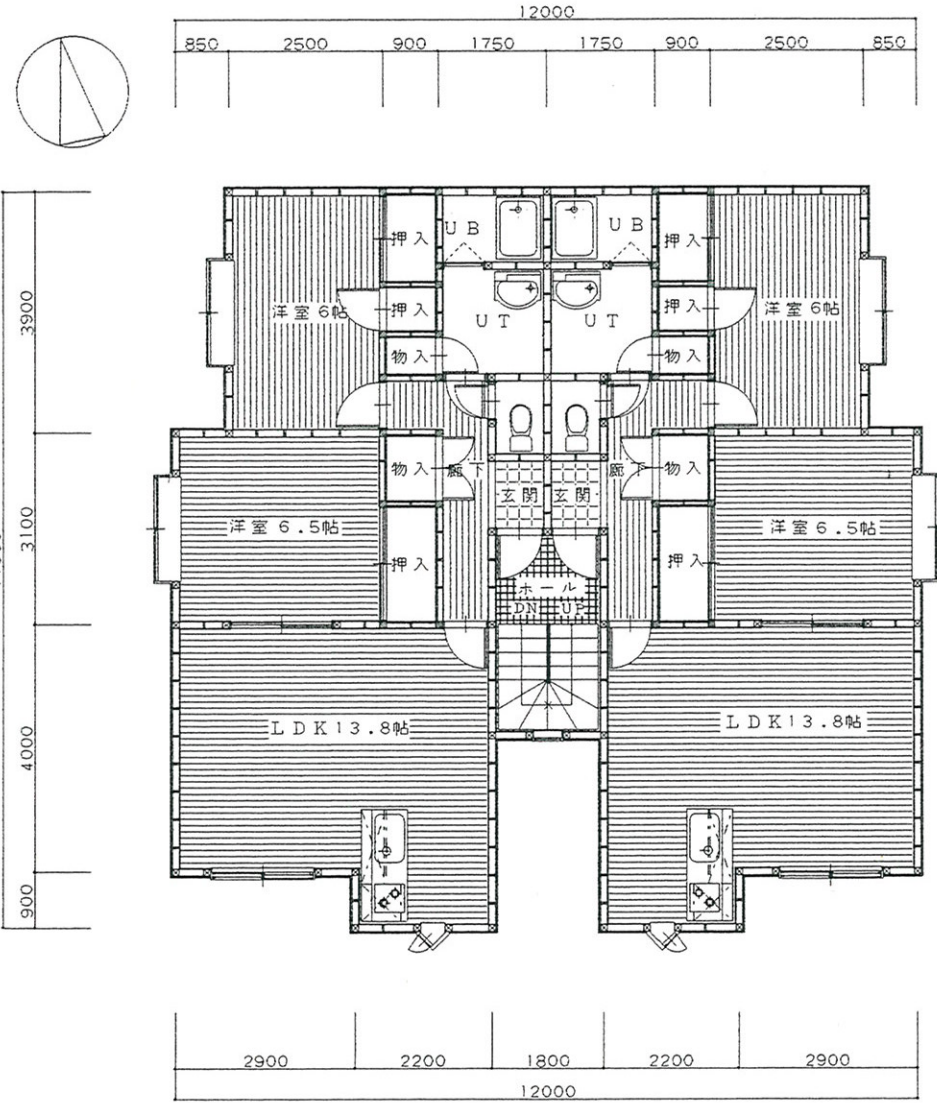
2.3階平面図
