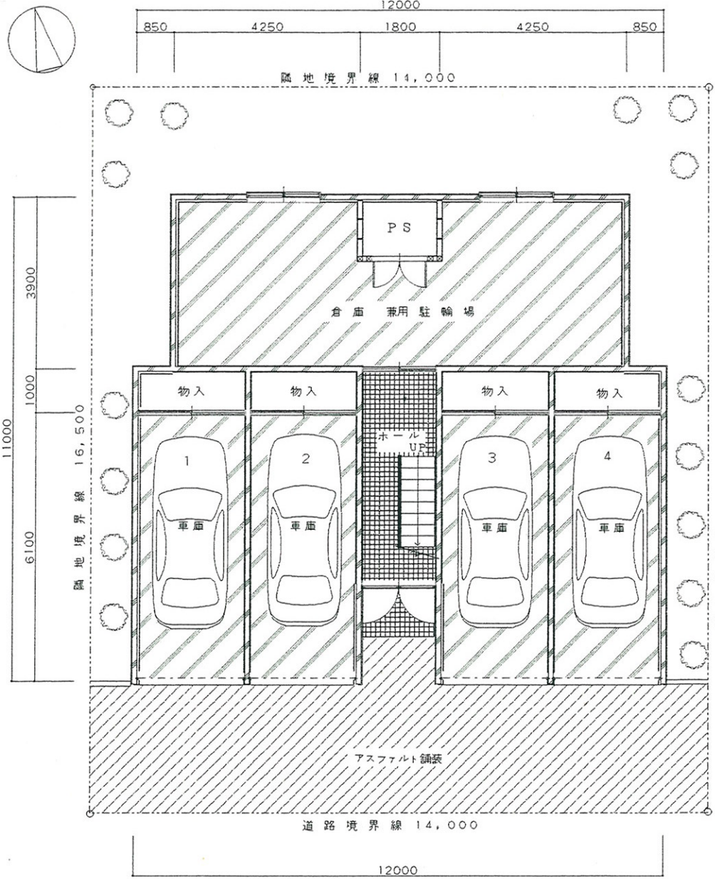
配置図 1階平面図
