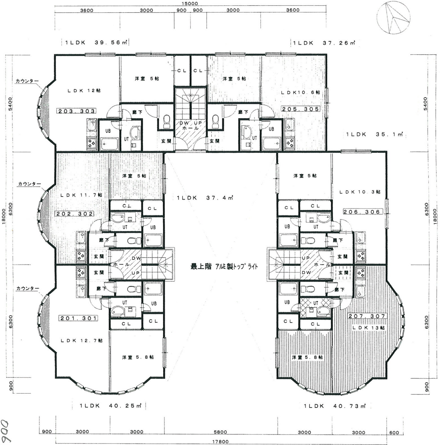
2. 3階 平面図
